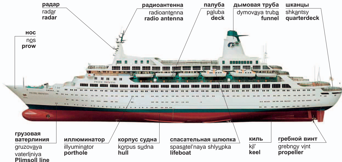
океанский лайнер okeanskiy layner | ocean liner
